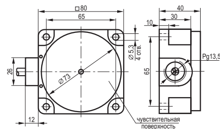
Габаритный чертеж
